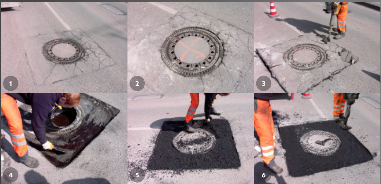
Regulierungen/Asphalteinbau
